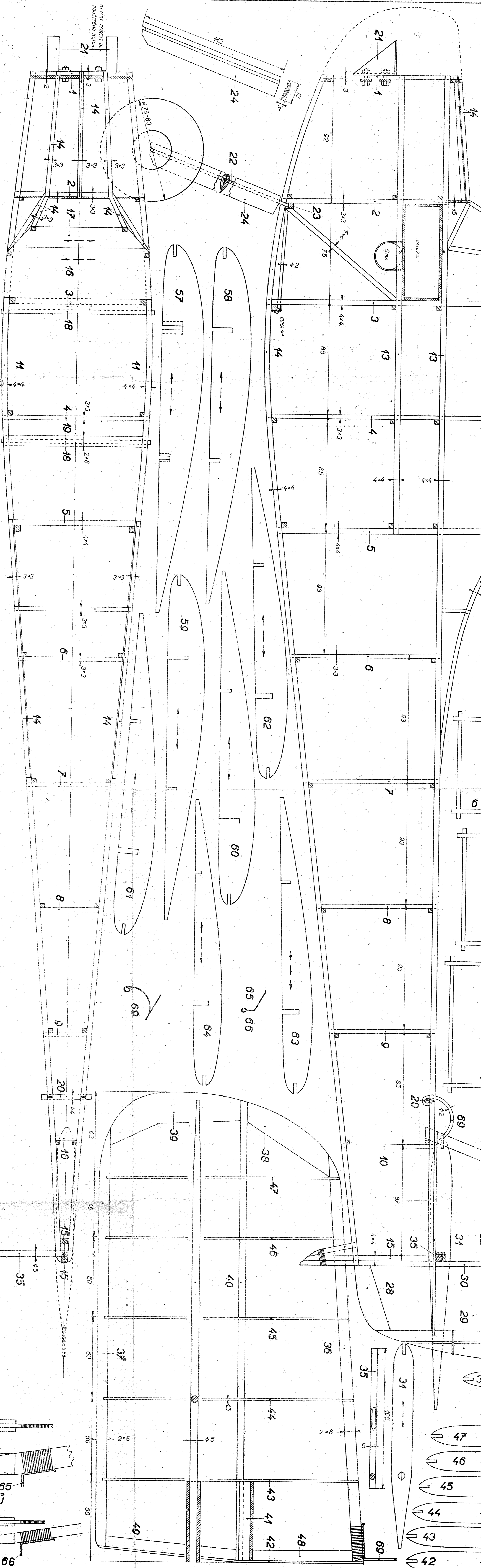
POHLED NA TRUP SE STRANY
